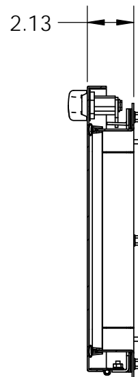
SECTION A-A SCALE 1 : 6
